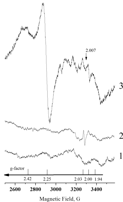
Рис. 1. Приклади спектрів ЕПР ТП, взятої на відстані 5 см від МВ ( a ); ТП, яка оточує МВ ( б ); тканини МВ ( в ). Спектри 1, 2 — розмір МВ < 5 мм; 3, 4 — розмір МВ > 1 см
