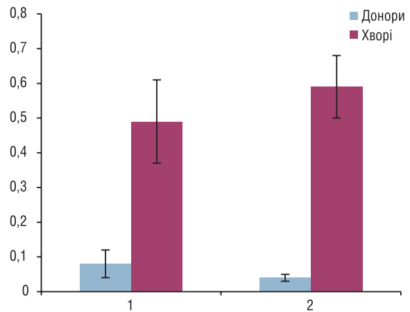
Рис. 4. Супероксид- (нМ/10 5 клітин·хв) та NO- (нМ/10 5 клітин) генеруюча активність нейтрофілів крові у хворих на мКРР: 1 — рівень СР; 2 — рівень NO
